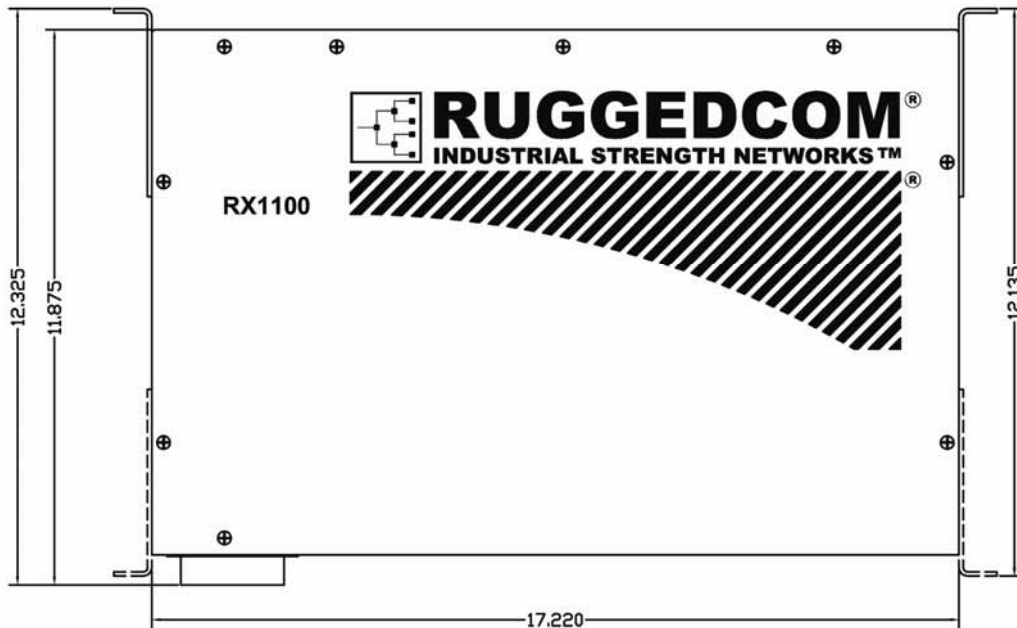
Вид сверху
