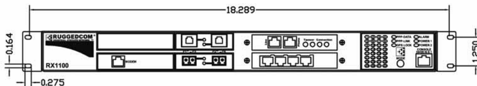
Вид спереди
