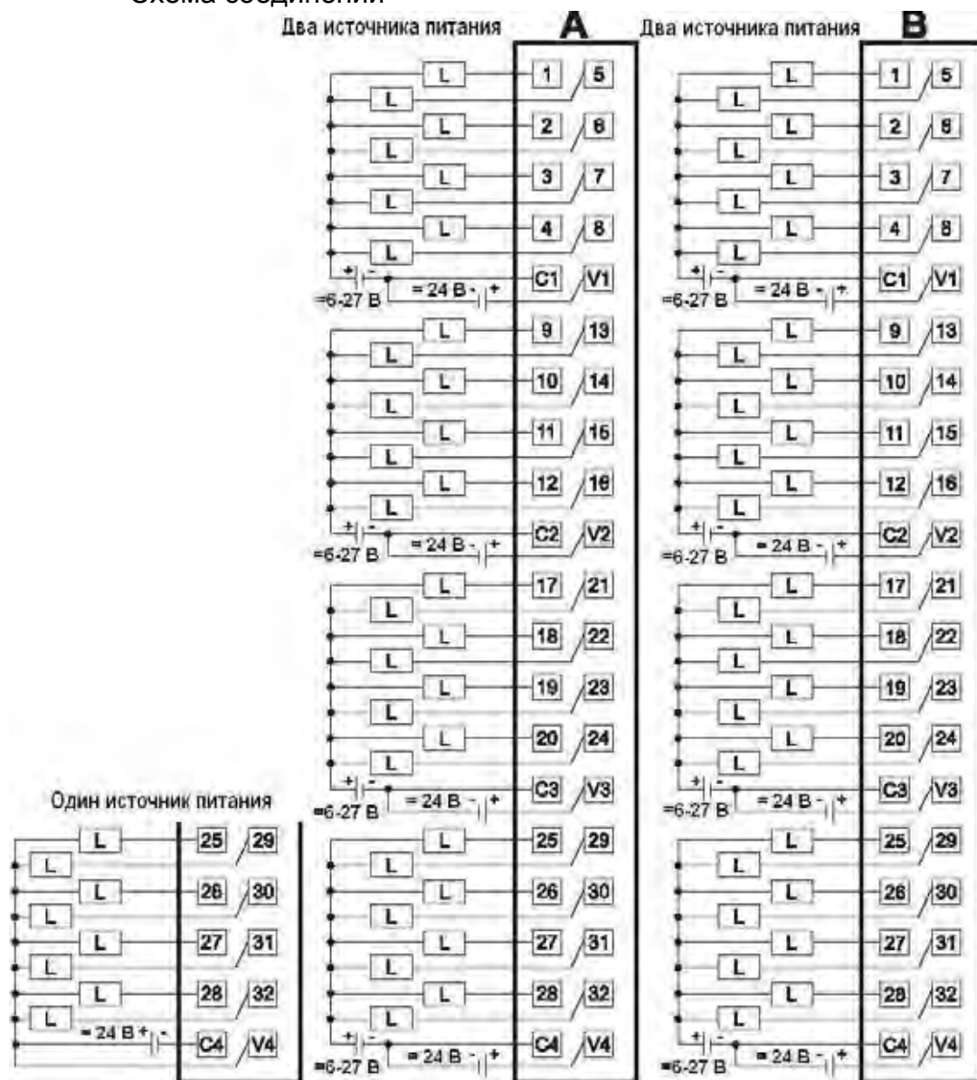
Схема соединений
