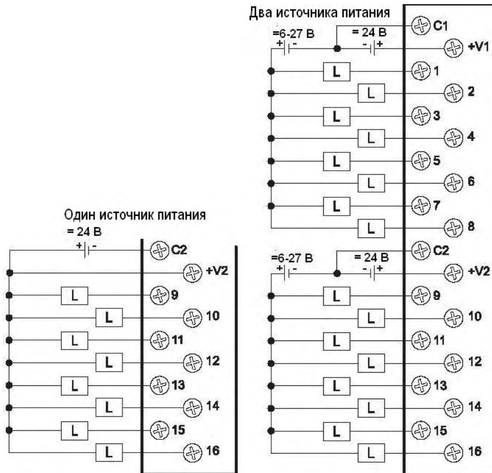
Схема соединений
