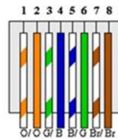
T-568B
