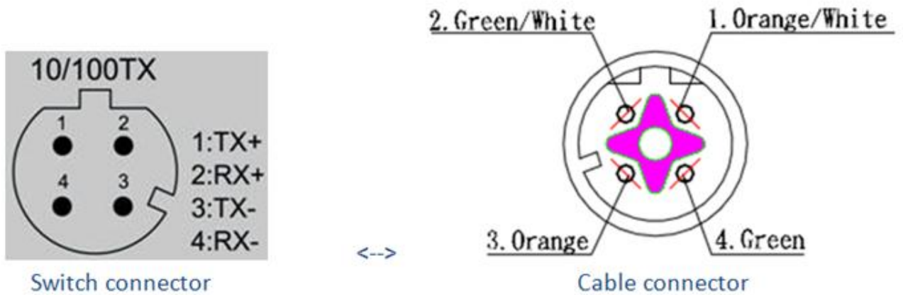
T-568B
