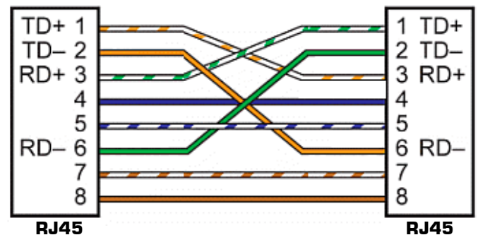
Перекрестный кабель 10BASE-T/100BASE-TX
