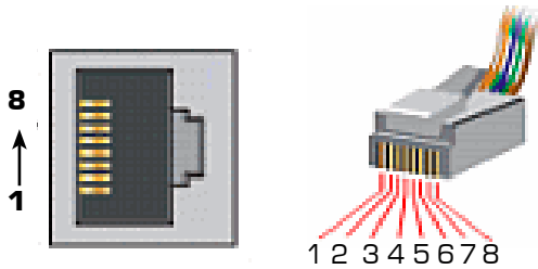
8-контактный RJ45 разъем (8P8C)
