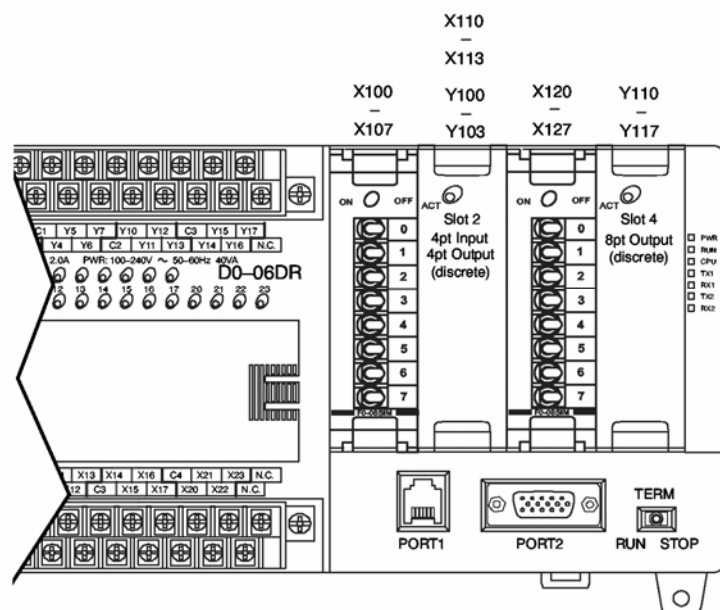
Пример адресации каналов модуля F0-08SIM
