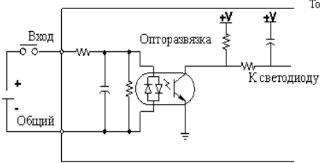
Эквивалентная схема входа Стандартные входы (X3-X7)
