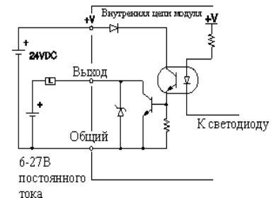
Эквивалентная схема выхода
