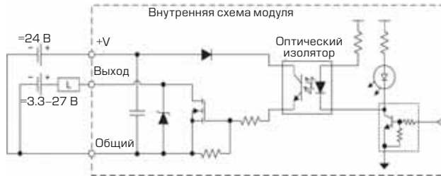
Эквивалентная схема выходов
