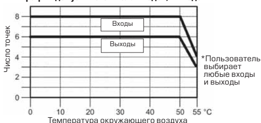
График допустимого числа входов/выходов
