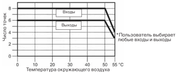
График допустимого числа входов/выходов
