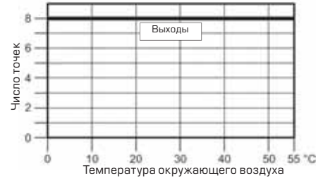
График допустимого числа выходов
