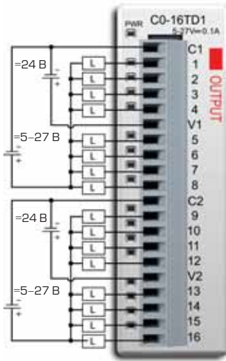
Эквивалентная схема выходов
