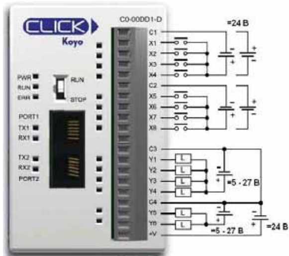
Эквивалентная схема входов
