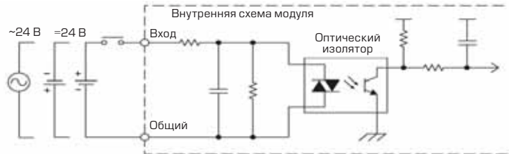
Эквивалентная схема входов
