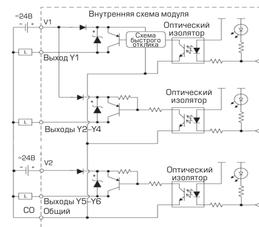
Эквивалентная схема выходов
