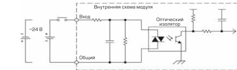
Эквивалентная схема входов
