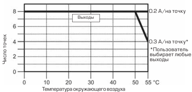
График допустимого числа выходов
