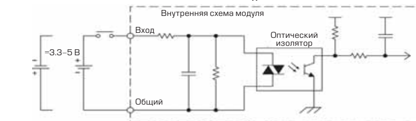
Эквивалентная схема входов
