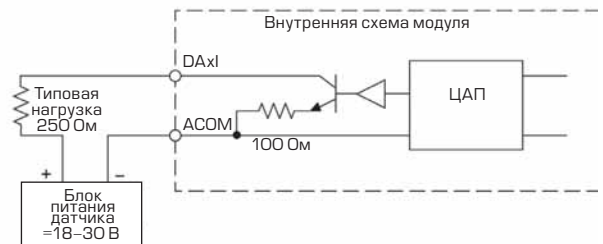
Схема аналогового токового выхода
