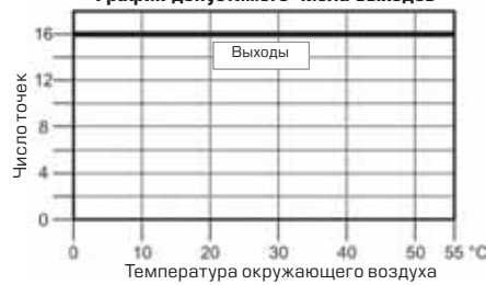
График допустимого числа выходов
