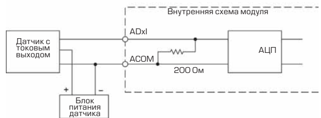
Схема аналогового токового входа
