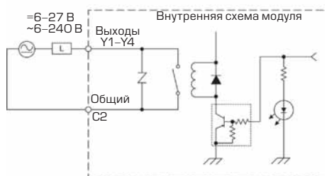
Эквивалентная схема выходов
