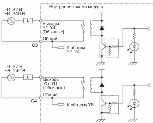
Эквивалентная схема выходов
